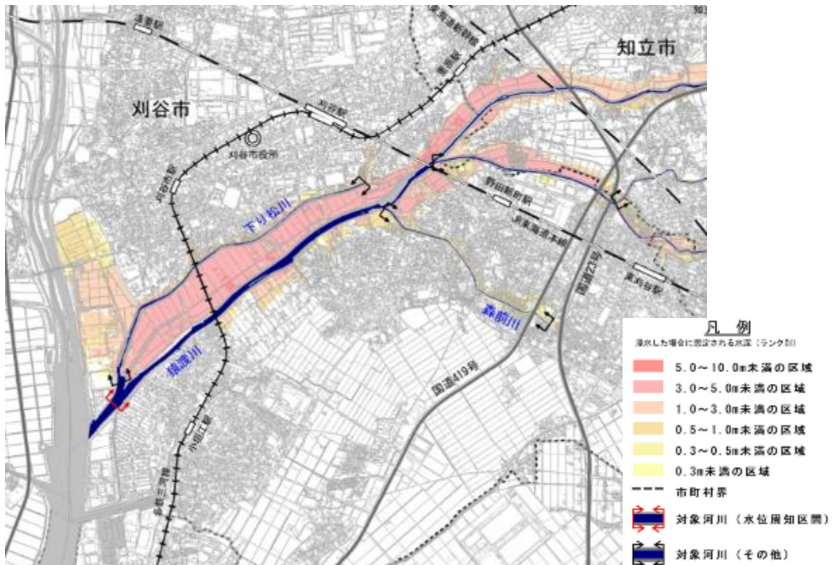
図 猿渡川流域 洪水浸水想定区域図（想定最大規模）（令和6年）
