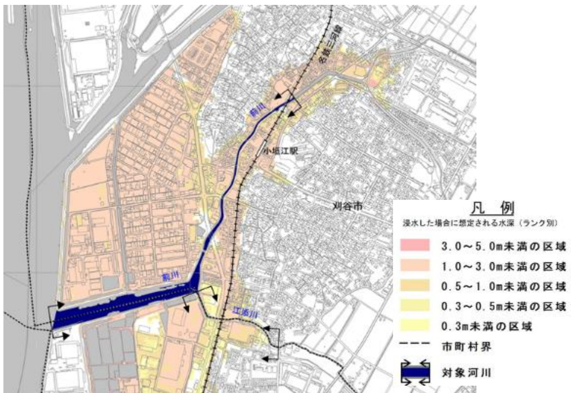
図 前川流域 洪水浸水想定区域図（想定最大規模）（令和6年）
