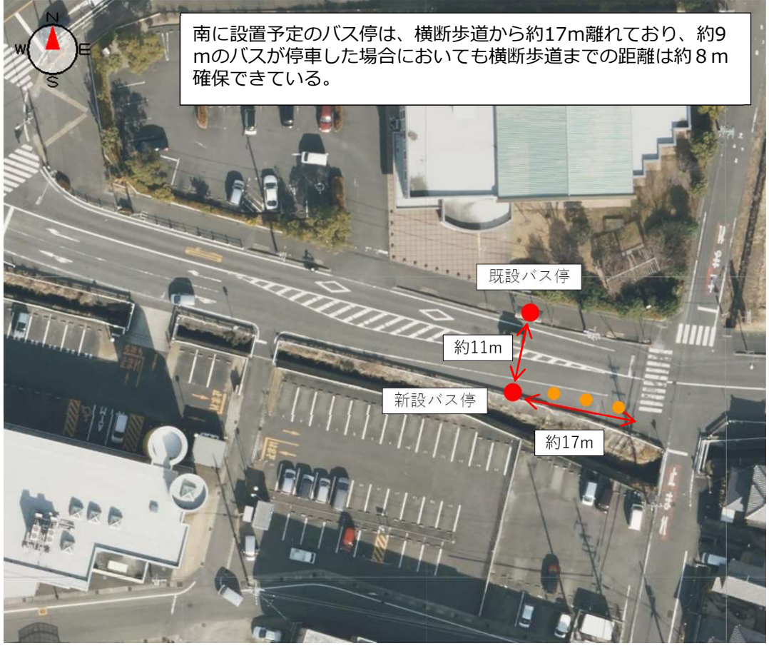
○平面図
