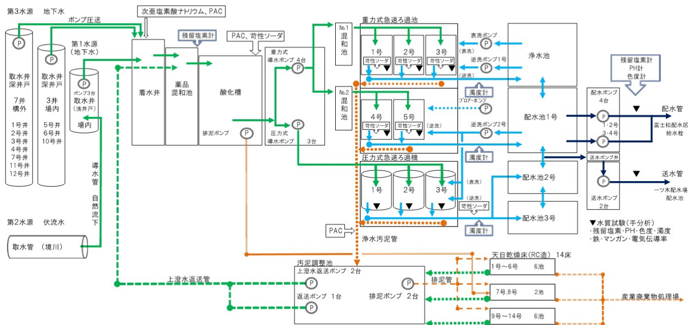
水源浄水場フロー図
