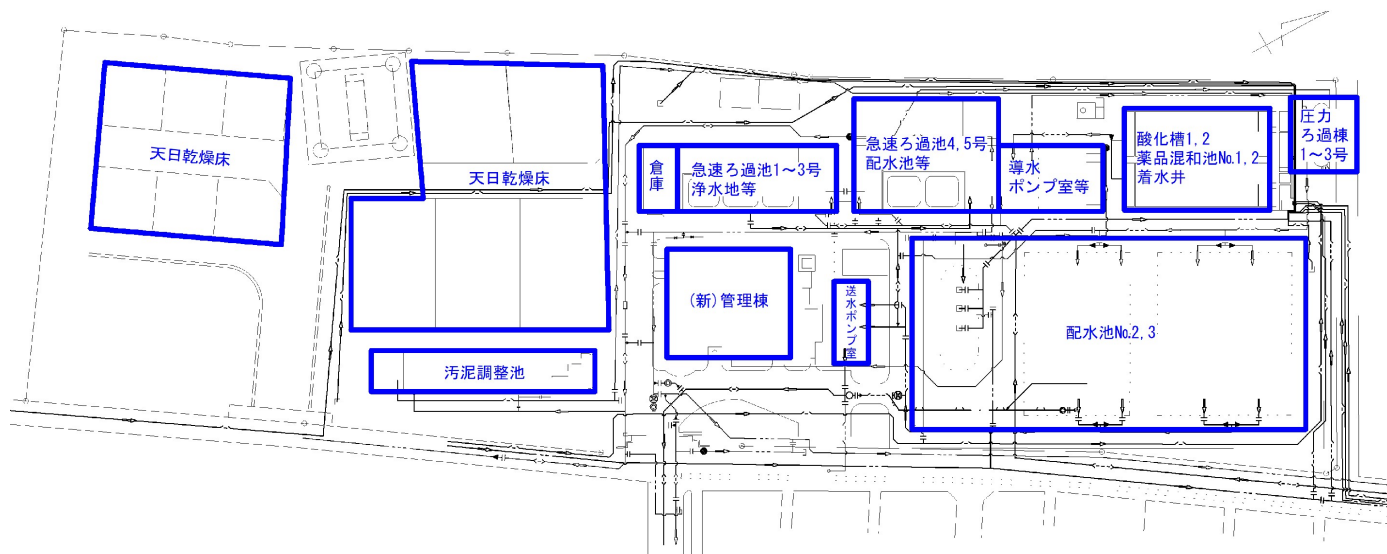
図4 既存浄水場平面図
