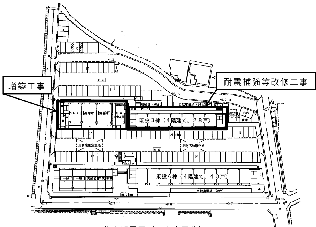
住宅配置図（工事完了後）
