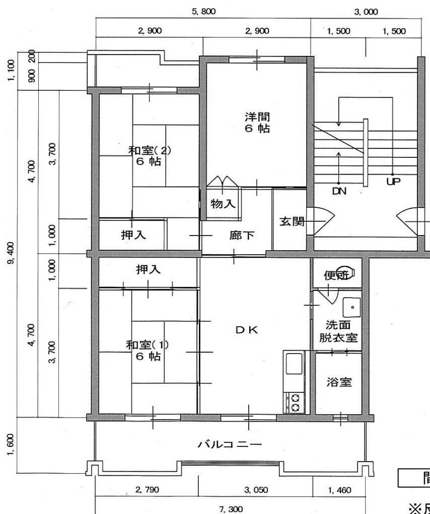
間取り図
