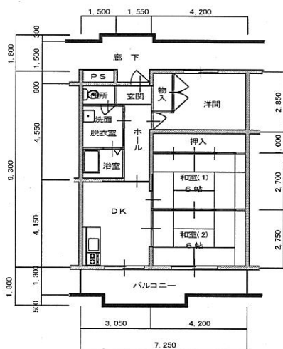
A・B棟 (2DK)
