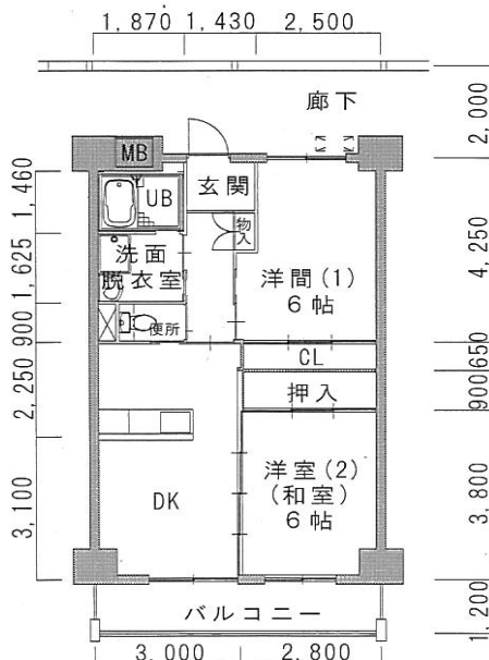
一般 2DK
