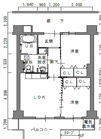
4棟(2LDK身障者用)
