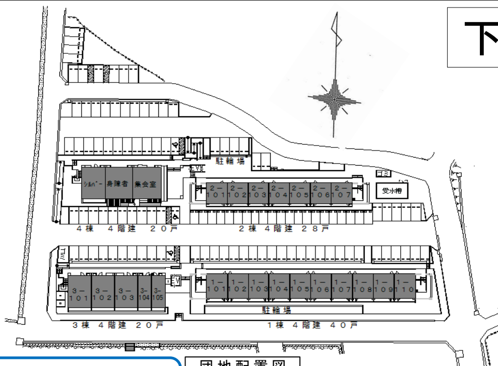
団地配置図
