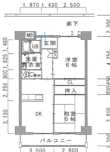
高齢者向 2DK
