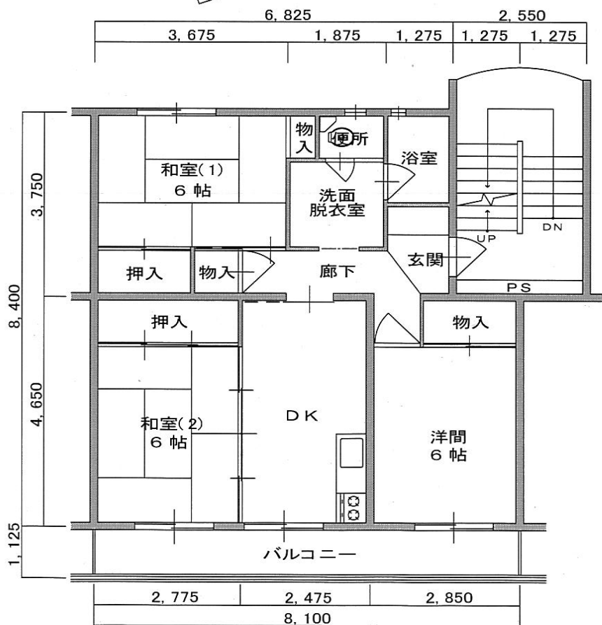
間取り図
