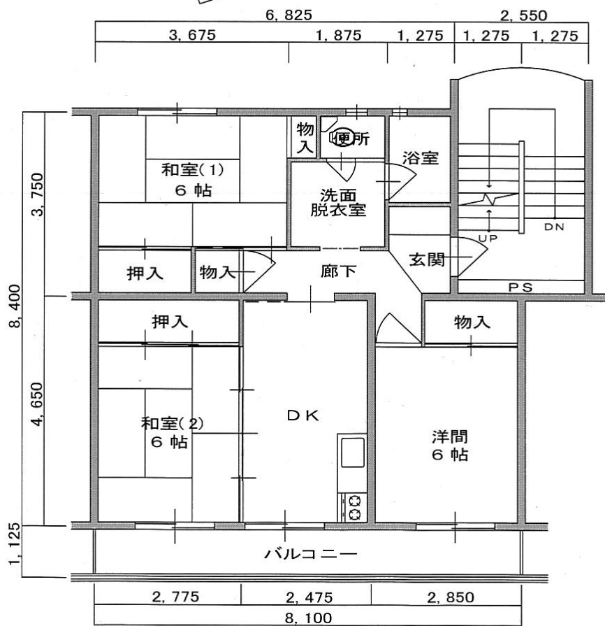
間取り図 ※反転タイプも有ります
