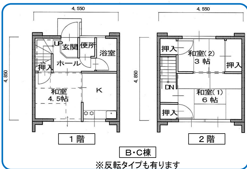
間取り図
