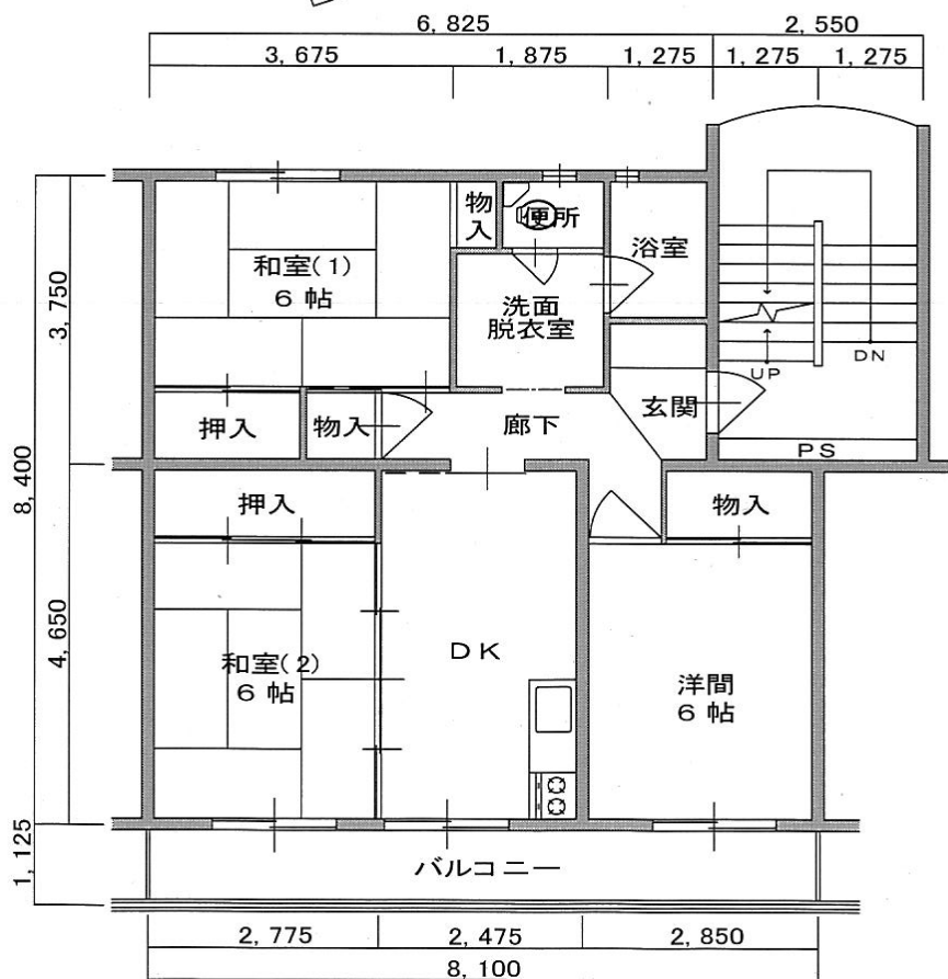
間取り図
