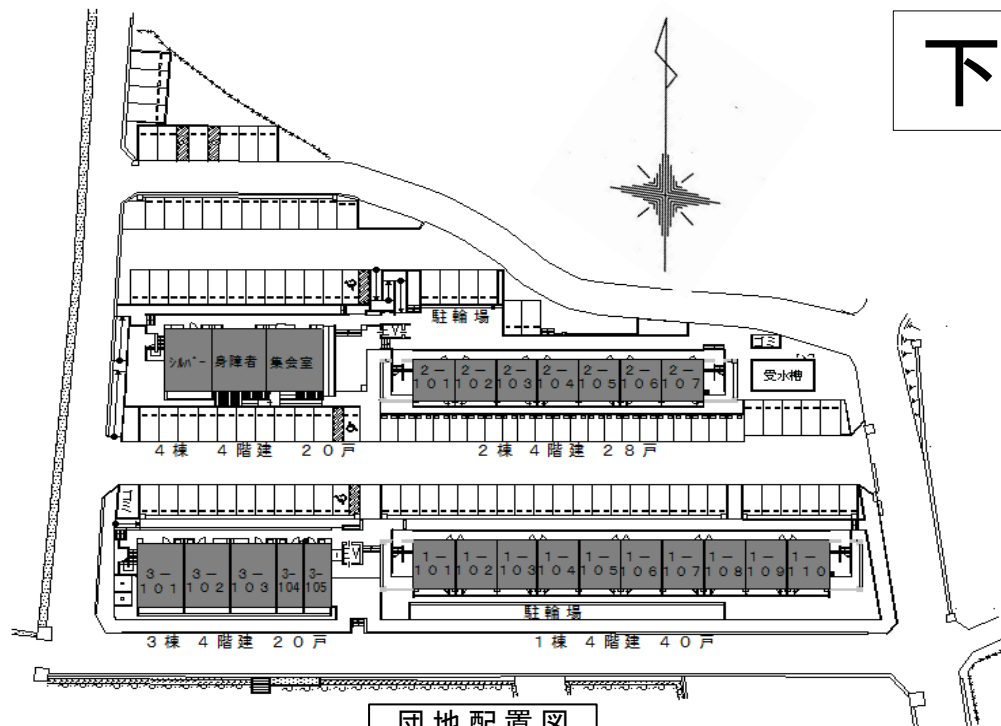
団地配置図
