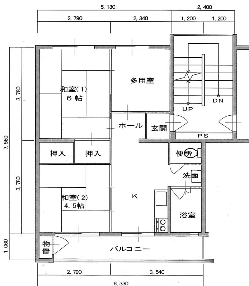
間取り図
