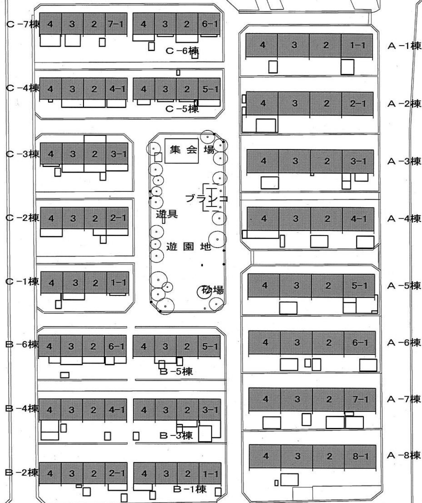
団地配置図
