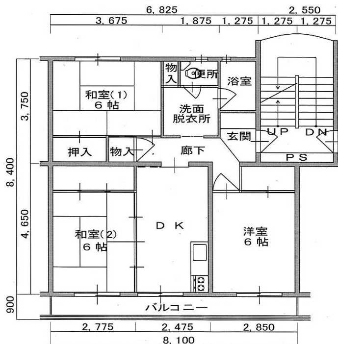
C・D棟
