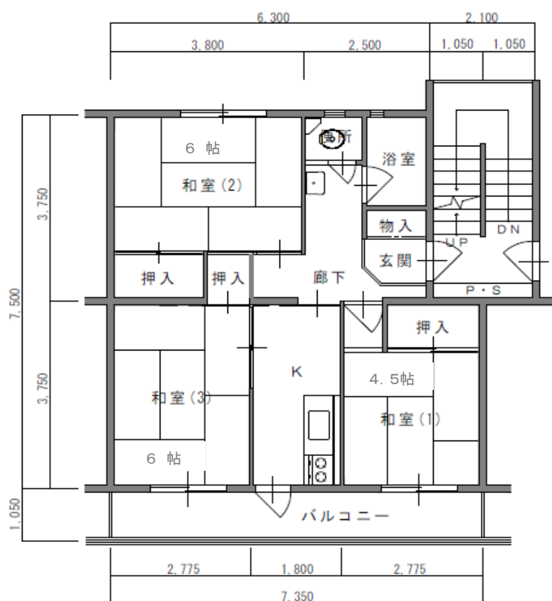
間取り図
