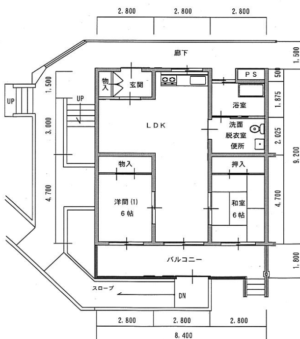
D棟(2LDK)身障者向
