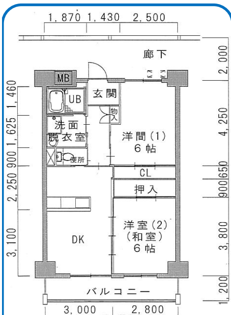
一般 2DK
