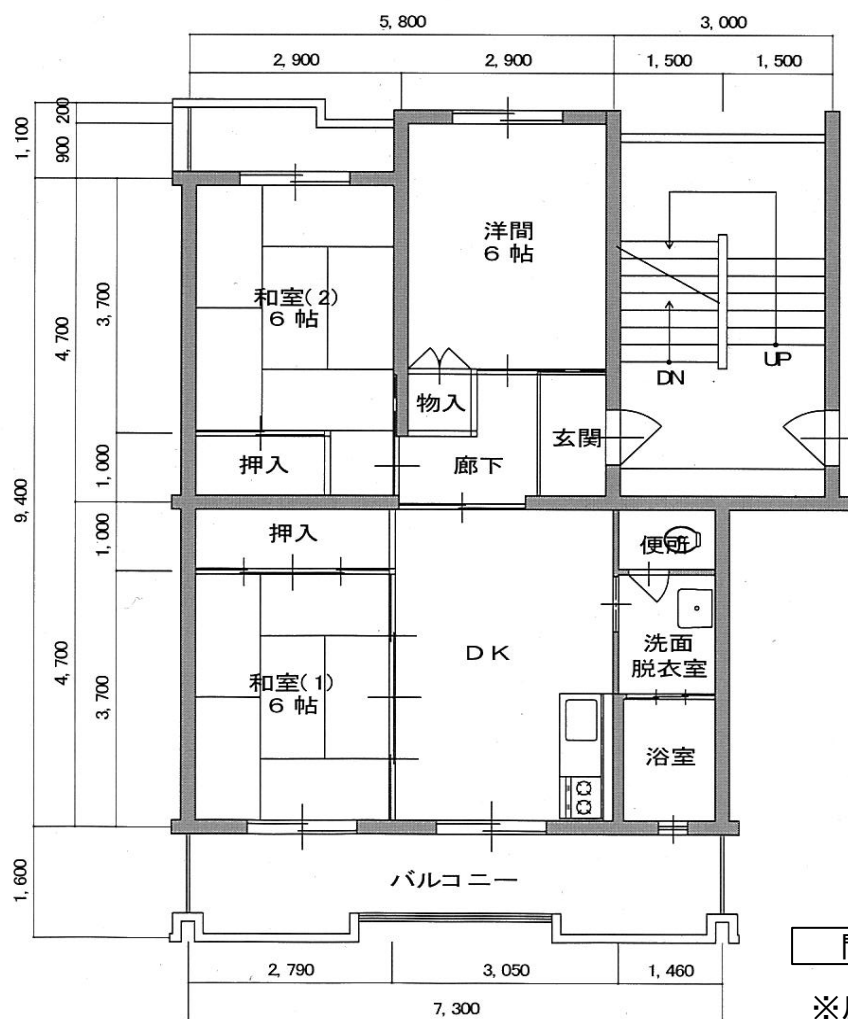
間取り図
